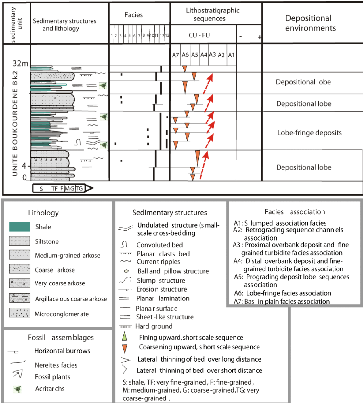
Figure 3: Analyse sédimentologique de l'unité sédimentaire 2 de Boukourdène (BK2). Figure 3. Sedimentological analysis of the Boukourdene sedimentary unit 2 (BK2).
