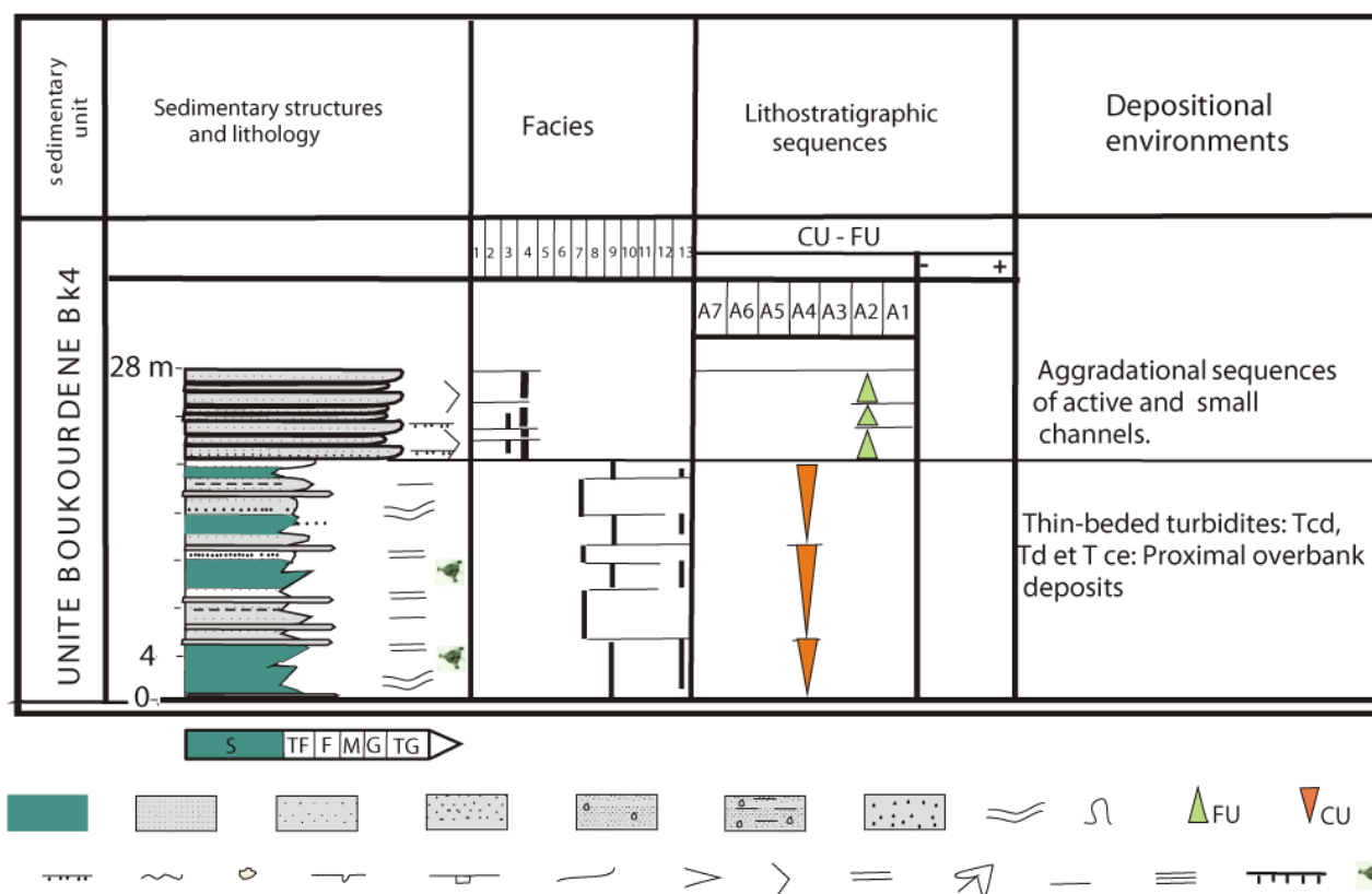
Figure 5: Analyse sédimentologique de l'unité sédimentaire 4 de Boukourdène, BK4 (légende, voir Fig. 3). Figure 5. Sedimentological analysis of the Boukourdene sedimentary unit 4, BK4 (legend, see Fig. 3).
