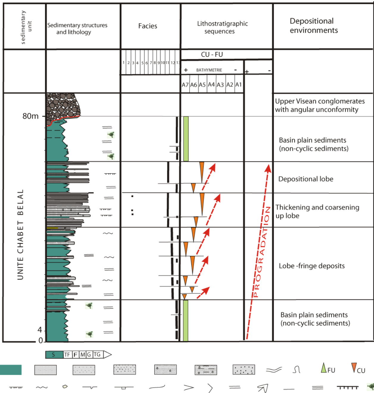
Figure 7: Analyse sédimentologique de l'unité sédimentaire de Chabet Belal, CHB (légende, voir Fig. 3). Figure 7. Sedimentological analyses of the Chabet Belal sedimentary unit, CHB (legend, see Fig. 3).
