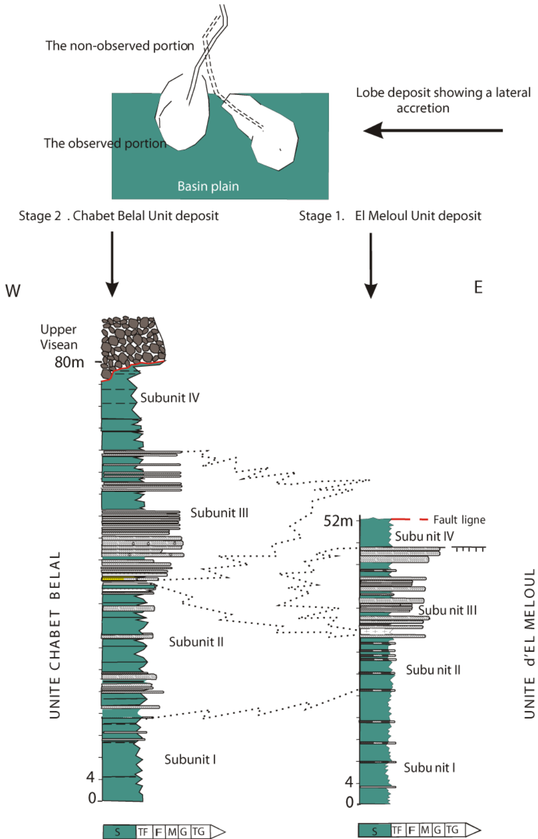
Figure 9: Modèle environnemental : Comparaison entre les unités sédimentaires de Chabet Belal-EI Meloul, les épaisseurs évoluent selon une polarité Est-Ouest. Figure 9. Environmental model: Comparison between the Chabet El Belal sedimentary unit and the Meloul sedimentary unit, the thicknesses are increasing according an east-west polarity.
