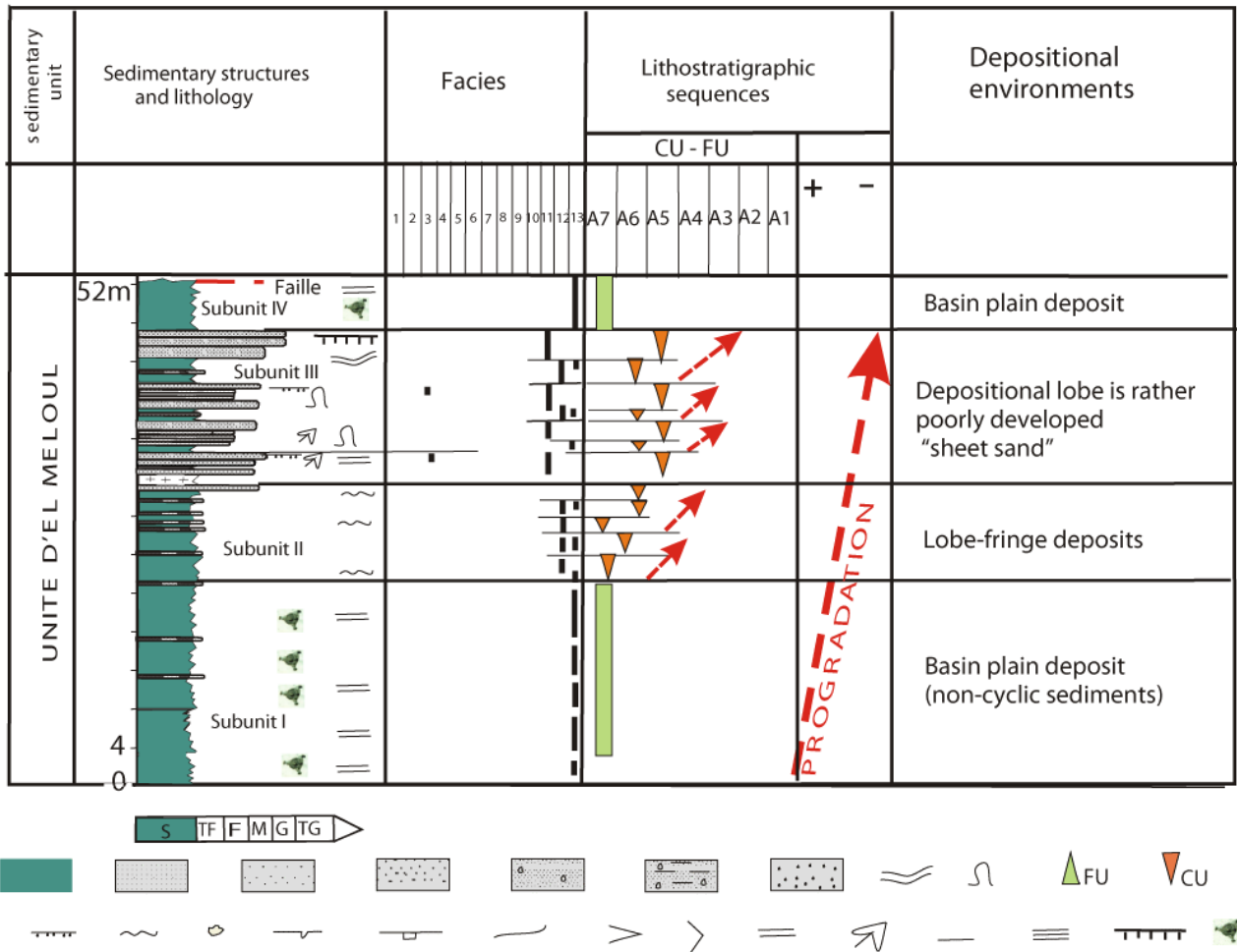
Figure 8: Analyse sédimentologique de l'unité sédimentaire d'El Meloul (légende, voir Fig. 3). Figure 8. Sedimentological analysis of the El Meloul sedimentary unit (legend, see Fig. 3).
